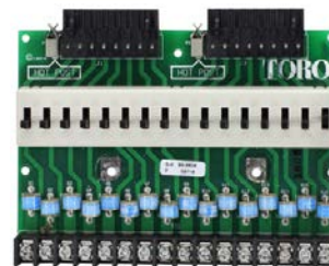
R102-8390 * Can also be used on VP & VPE / Également utilisé pour VP & VPE M4 Surge Board (Lead Free)
